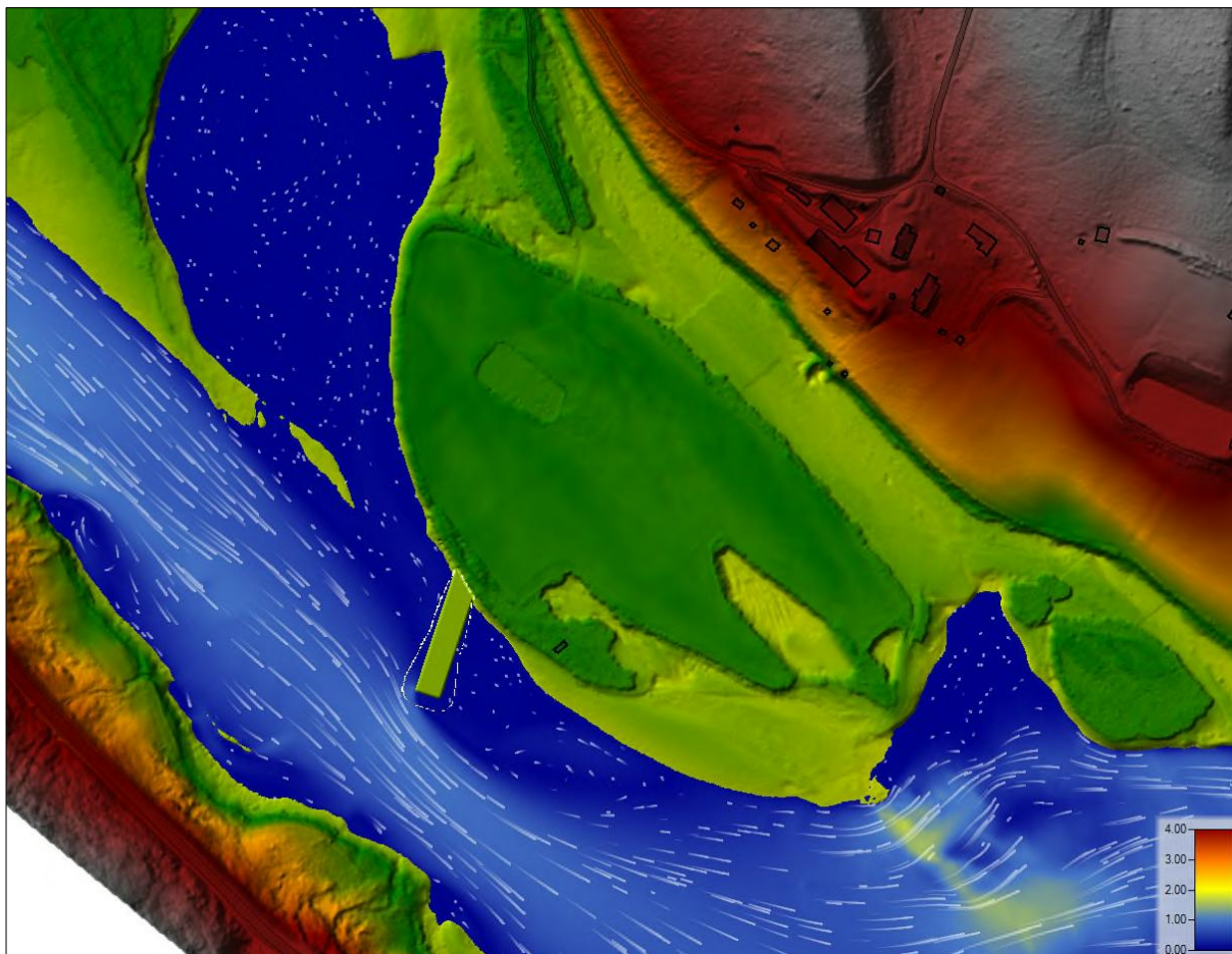
Figur 74. Anleggsfase justert løsning, hastighet og strømningsretninger, Q_{20} i vinterperiode i Lågen og median vannstand i Mjøsa (blå farge viser lave hastigheter, mens rød/ oransje farge høye hastigheter).
