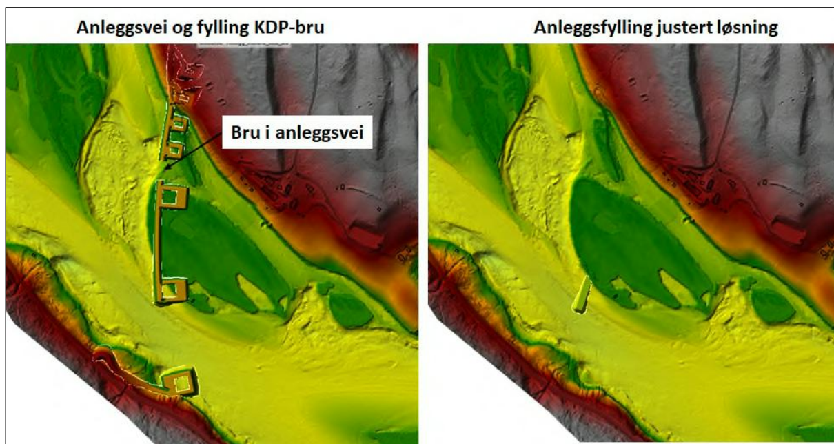
Figur 68. Anleggsfase, terrengmodell
