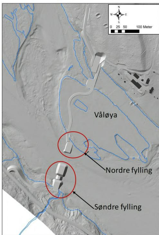
Figur 68. Anleggsfase, terrengmodell
