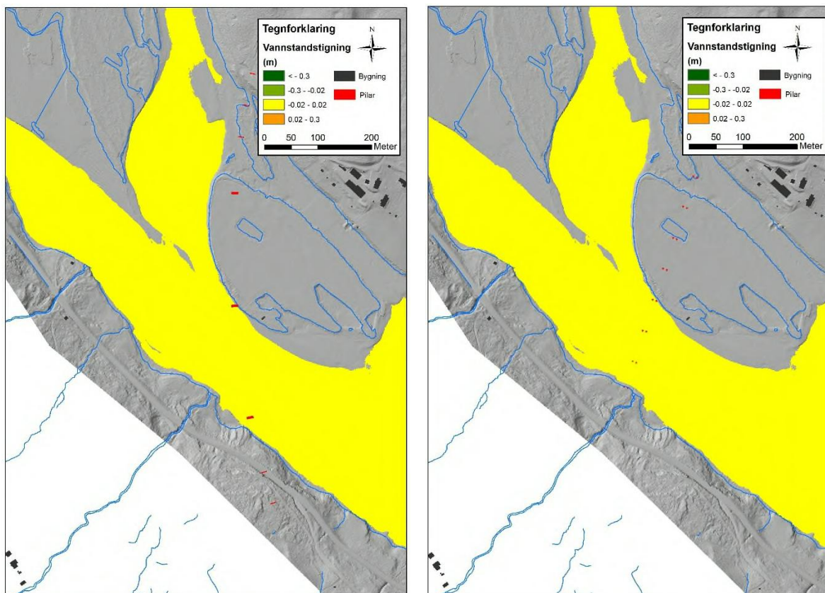
Figur 75. Visualiseringer viser vannstandsendringer medført av Fritt frambygget bru (venstre) og kassebru (høyre) i Lågendeltaet ved middelvannsføring ( Q_{\text{middel}} ) ved laveste regulerte vannstand på våren (april-mai).
